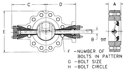
LUGGED
